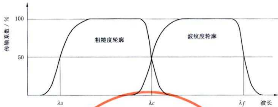
图1 粗糙度和波纹度轮廓的传输特性
