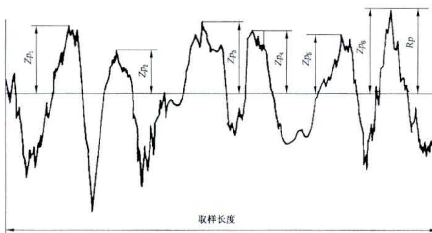
图 6 最大轮廓峰高(以粗糙度轮廓为例)
