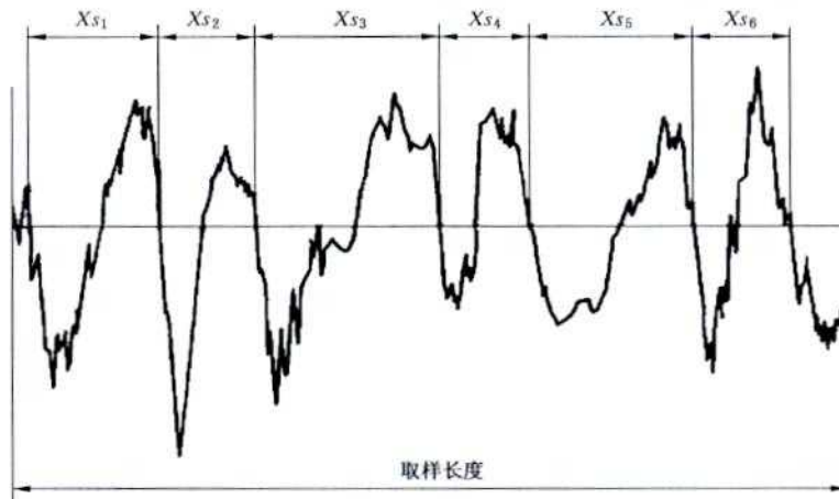
图10 轮廓单元的宽度
