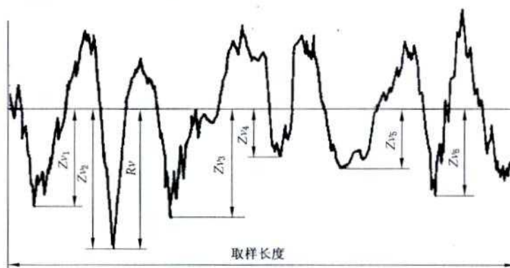
图 7 最大轮廓谷深(以粗糙度轮廓为例)
